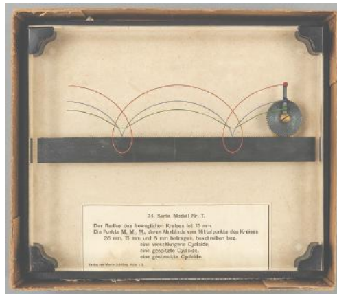
Ryc. 17 a–c. Modele kinematyczne M. Schillinga, seria XXIV, nr 5, 6 oraz 7, wł. Muzeum UJ, fot. G. Zygiel
